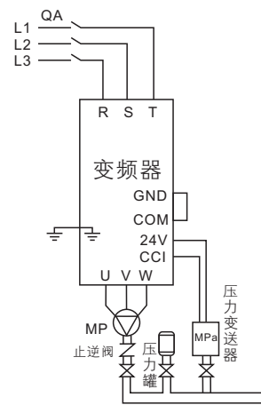
图5-1-1B 电流型压力传感器 (压力变送器, F9-03=1) (CCI跳线至4~20mA)
