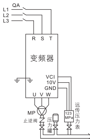
图5-1-1A 电压型压力传感器 (远传压力表, F9-03=0)
