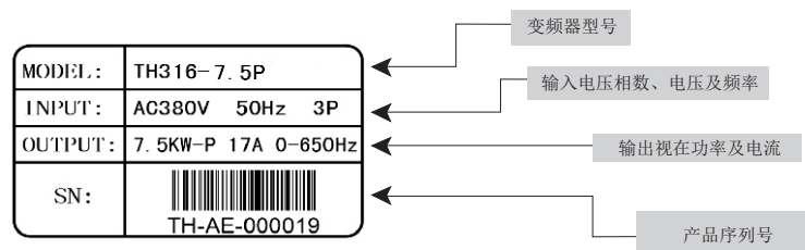
图1.1 铭牌示意图
